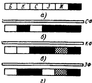
Рис. 19. Образование различных цветоделенных сигналов в телепередатчиках цветного телевидения.
