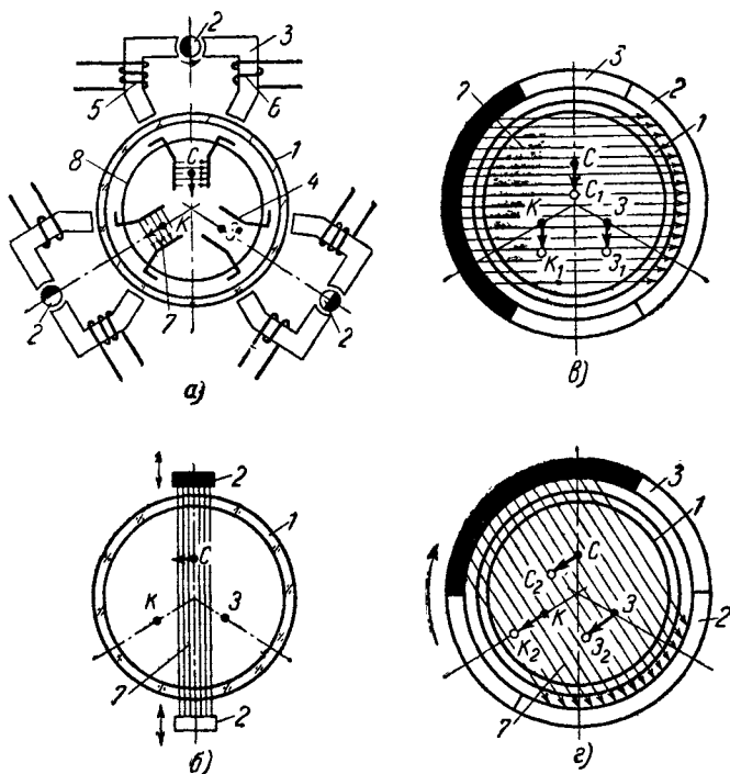
Рис. 22. Принцип действия магнитов корректировки. Вид от экрана.
