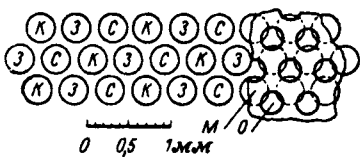
Рис. 20. Строение экрана цветного кинескопа с тневой маской. Вид изнутри кинескопа при сильном увеличении.
