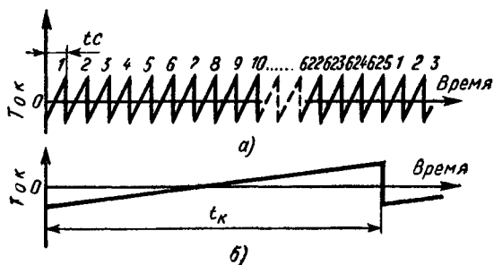
Рис. 10. Изменение во времени величины тока через катушки отклоняющей системы.
