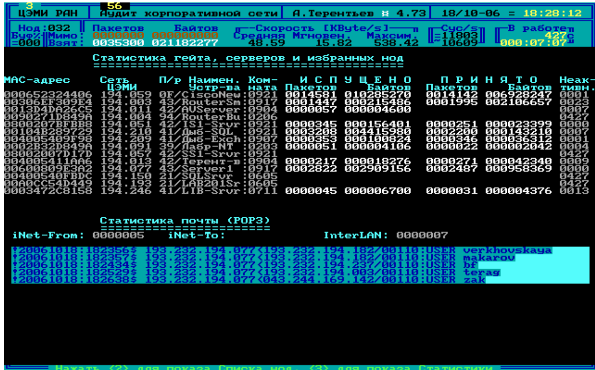
Рис. 14. Экран показа статистики выделенных серверов и почты «3»
