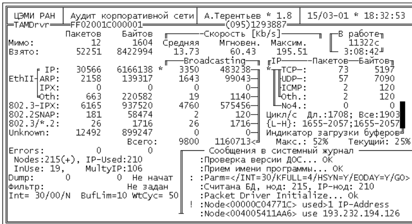
Рис. 10. Верхняя часть основного экрана программы наблюдения
